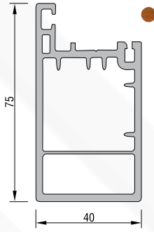
SASH PROFILE R 21601-01003 : ROBLE
